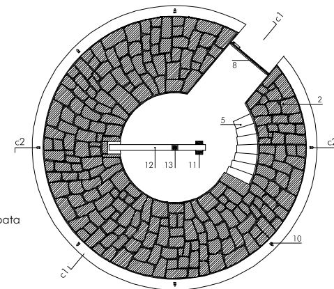
planta A
