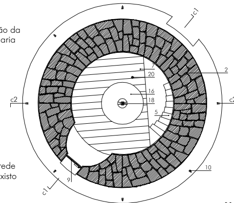
planta B
