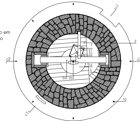
planta C
