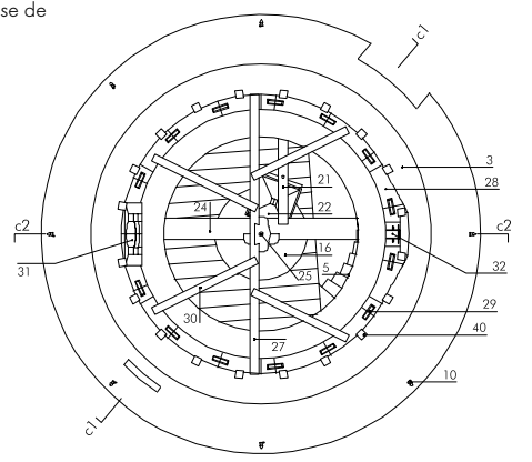
planta D
