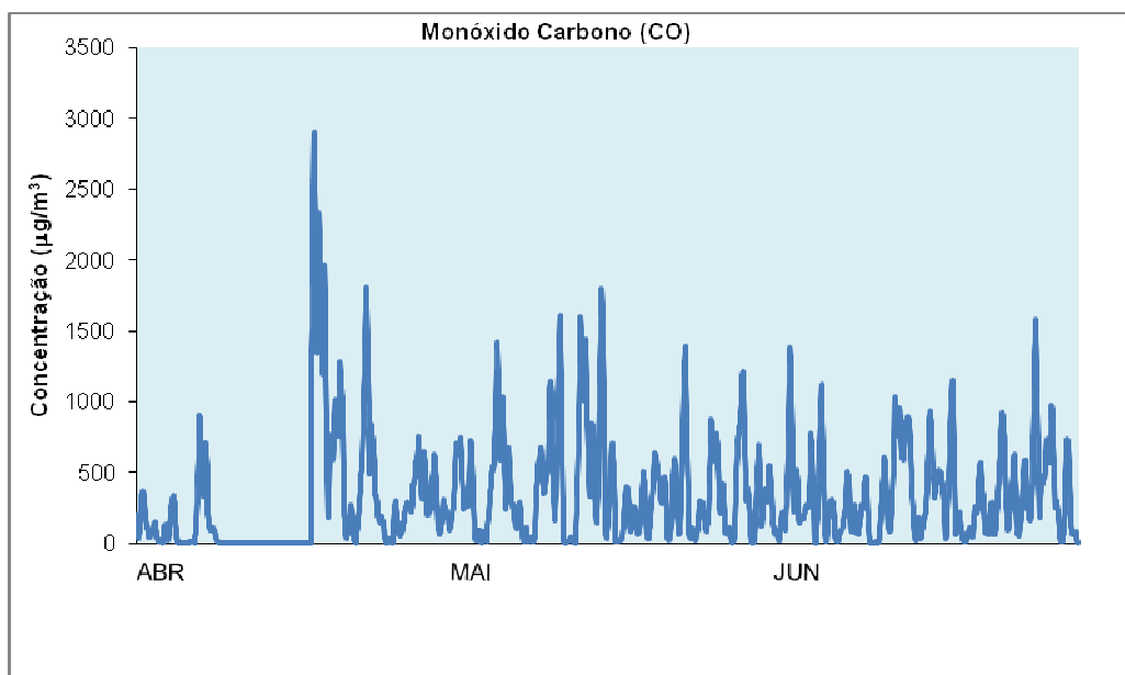
Gráfico 24 – Máximo diário das médias 8 horas das concentrações de CO – David Neto
