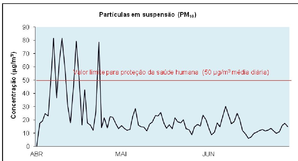
Gráfico 1 – Médias diárias das concentrações de PM 10 - Cerro
