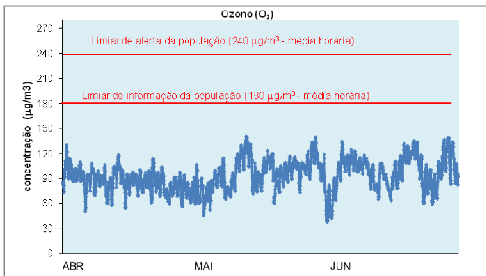
Gráfico 18 – Médias Horárias das concentrações de O 3 – Cerro
