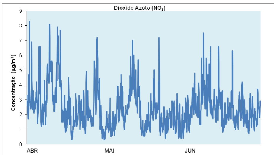
Gráfico 11 – Médias horárias das concentrações de NO 2 – Cerro
