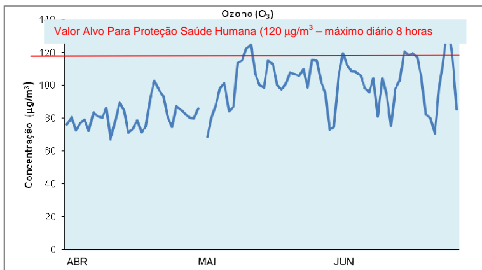
Gráfico 23 – Máximo das médias octo-horárias das concentrações de O 3 – Joaquim Magalhães
