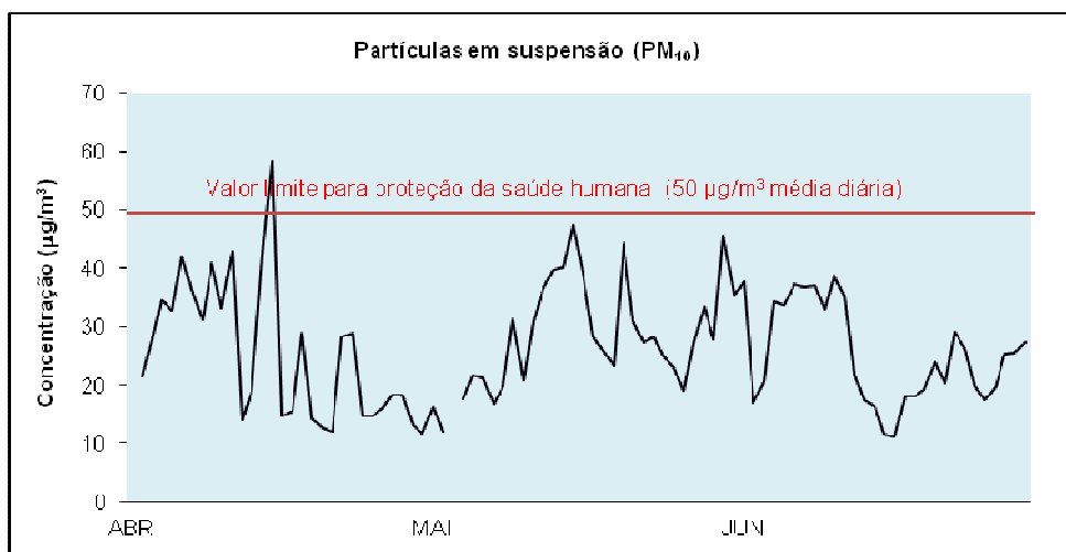
Gráfico 3 – Médias diárias das concentrações de PM 10 - Malpique
