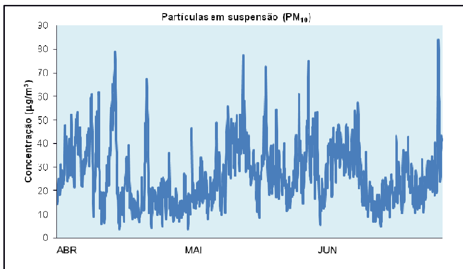
Gráfico 4 – Médias horárias das concentrações de PM 10 - Malpique
