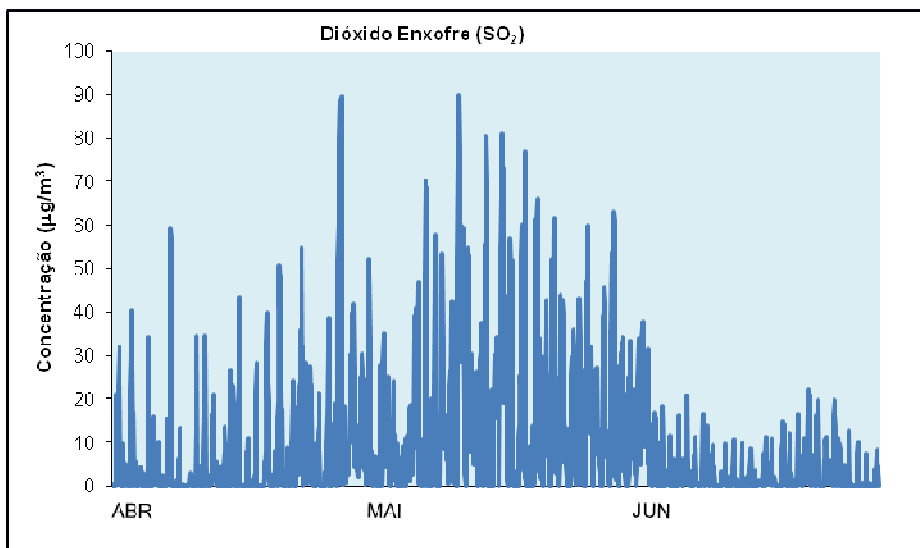
Gráfico 14 – Médias horárias das concentrações de SO 2 – Cerro
