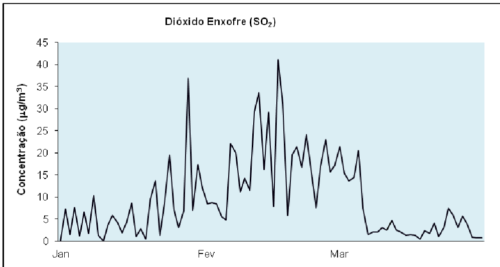
Gráfico 15 – Médias diárias das concentrações de SO 2 – Cerro
