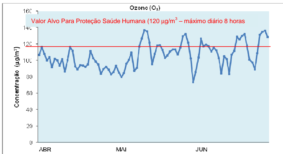
Gráfico 19 – Máximo das médias octo-horárias das concentrações de O 3 – Cerro
