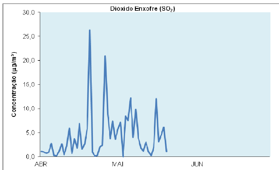
Gráfico 17 – Médias diárias das concentrações de SO 2 – Joaquim Magalhães
