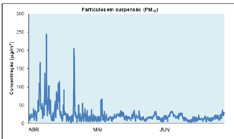
Gráfico 2 – Médias horárias das concentrações de PM 10 - Cerro
