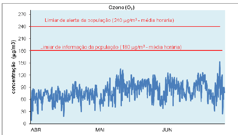
Gráfico 22 – Médias Horárias das concentrações de O 3 – Joaquim Magalhães
