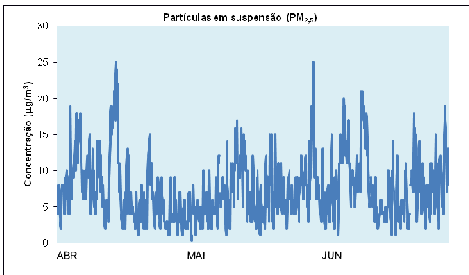
Gráfico 9 – Médias horárias das concentrações de PM 2,5 – Cerro
