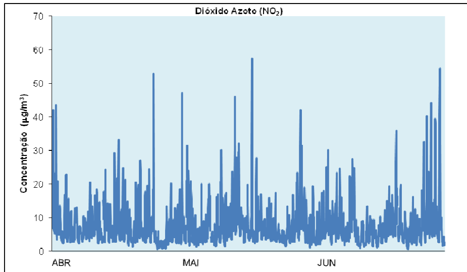
Gráfico 13 – Médias horárias das concentrações de NO 2 – Joaquim Magalhães
